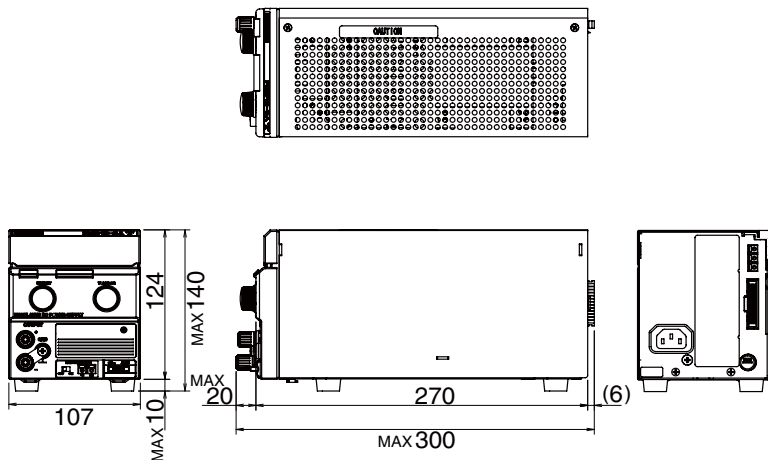
図 7-1 PMC-A タイプ I 外形寸法図 単位 : mm
