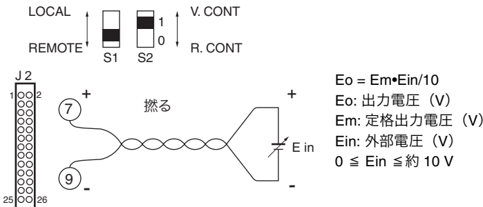
図 5-3 CV-V の設定および接続
