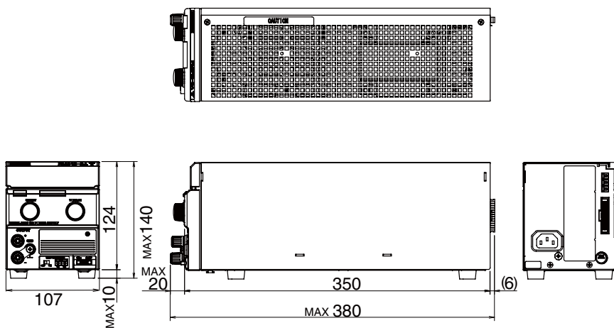
図 7-2 PMC-A タイプ II 外形寸法図 単位 : mm
